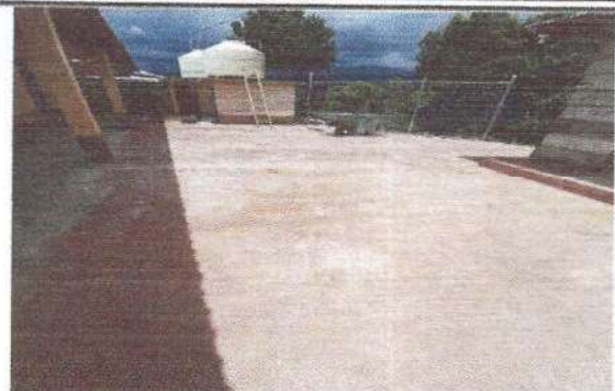
Foto 2: Finalización de la sustitución de piso de torta de concreto de 8 cm de espesor
